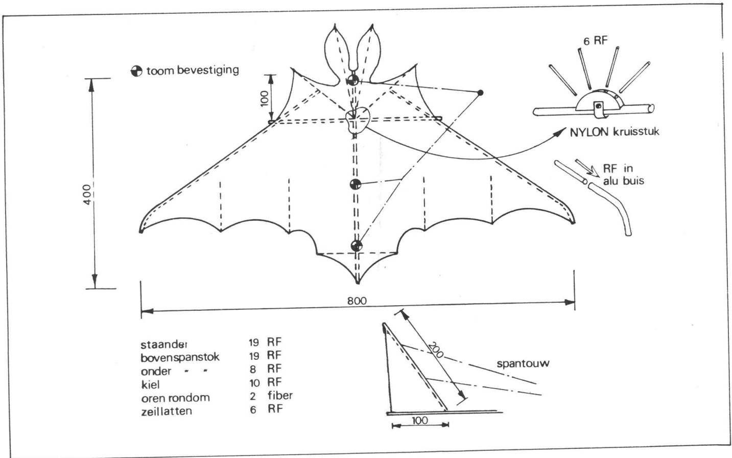
Staartkiel met spantouwen van de VLEERMUIS.
