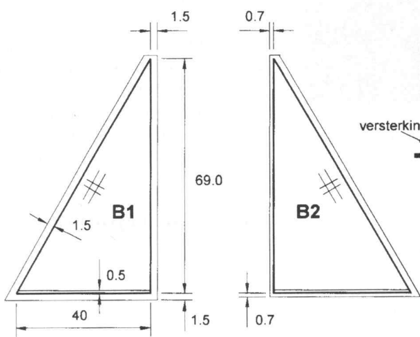
BUITENCELLEN 6X PANEEL B1 6X PANEEL B2
